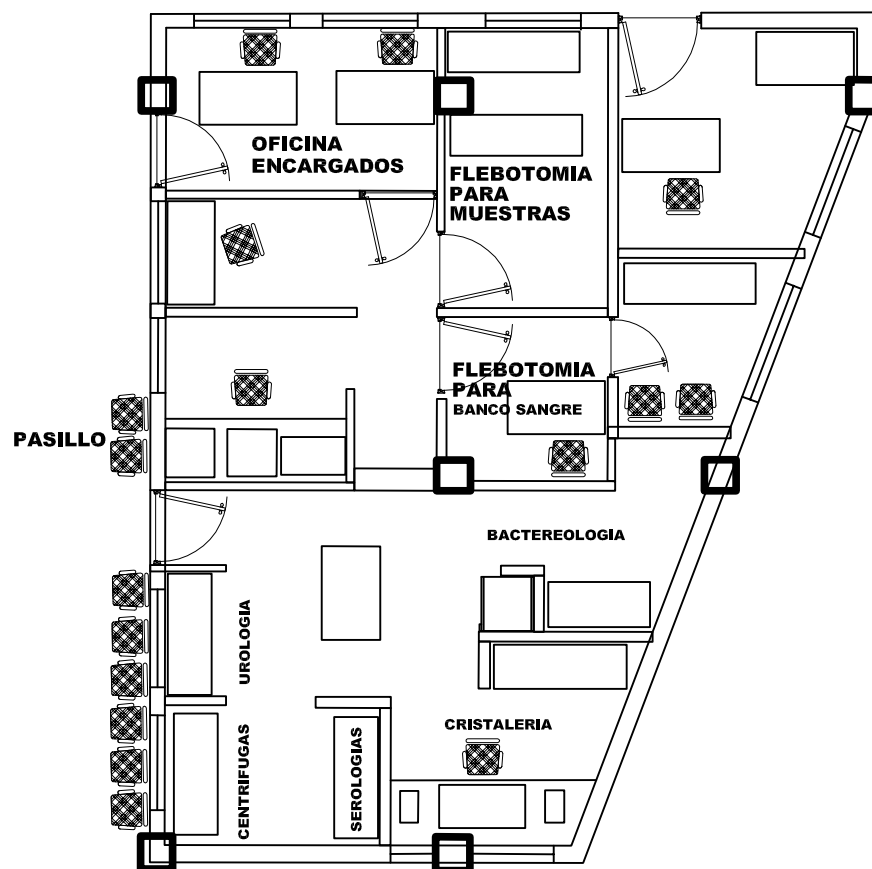
PLANTA ARQUITECTONICA DE PROYECTO: LABORATORIO DE HOSPITALITO SANTIAGO ATITLAN, SOLOLA.
