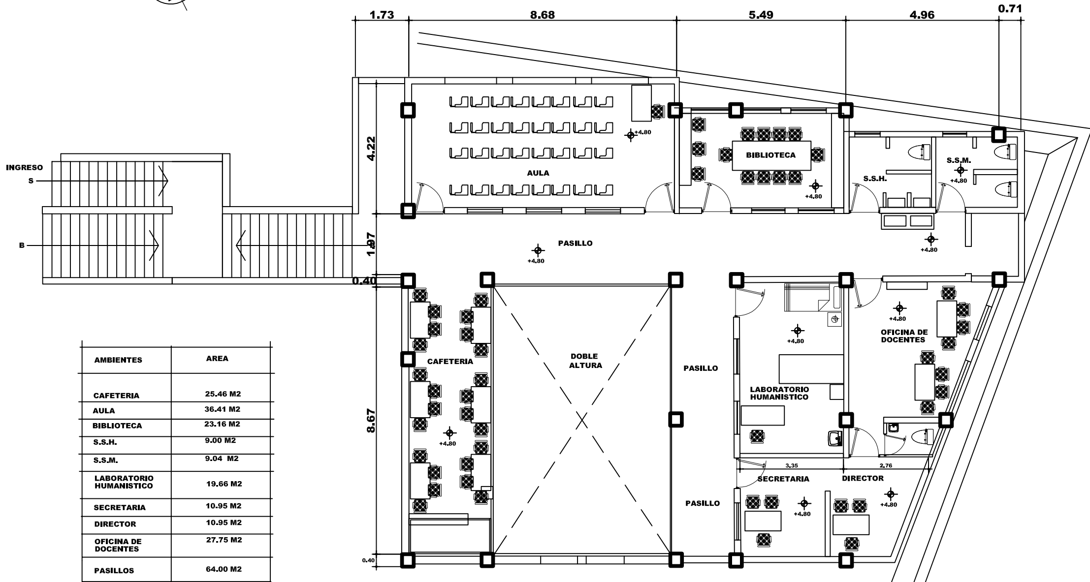
PLANTA ARQUITECTONICA DE PROYECTO: ESCUELA PRIVADA MAYA AUXILIAR DE ENFERMERIA SANTIAGO ATITLAN, SOLOLA.
